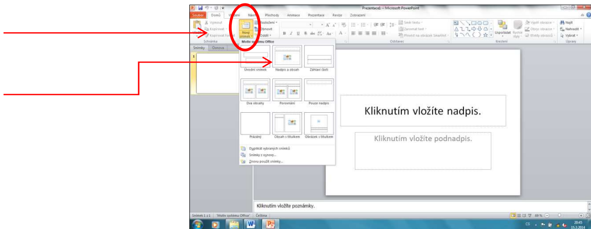
Obrázek 2 - rozložení snímku
