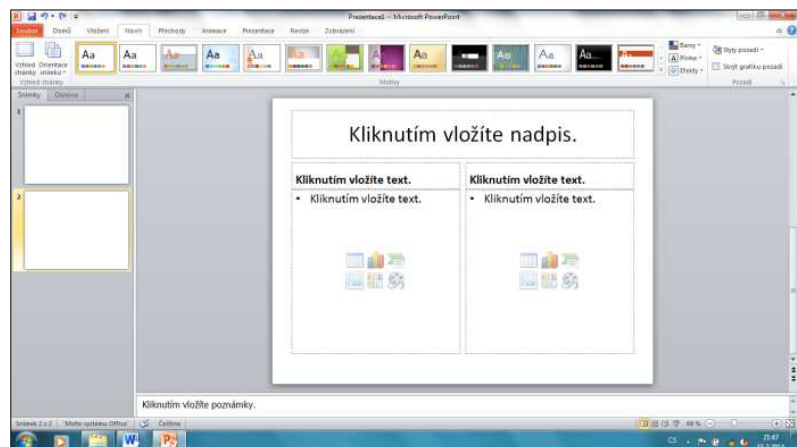
Obrázek 4 - pozadí snímků
